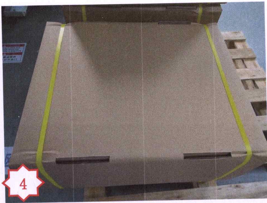
图四, 确认 PA3213 无漏装后, 将 26 的内箱与外箱配合, 并打包装带, 待出货。
